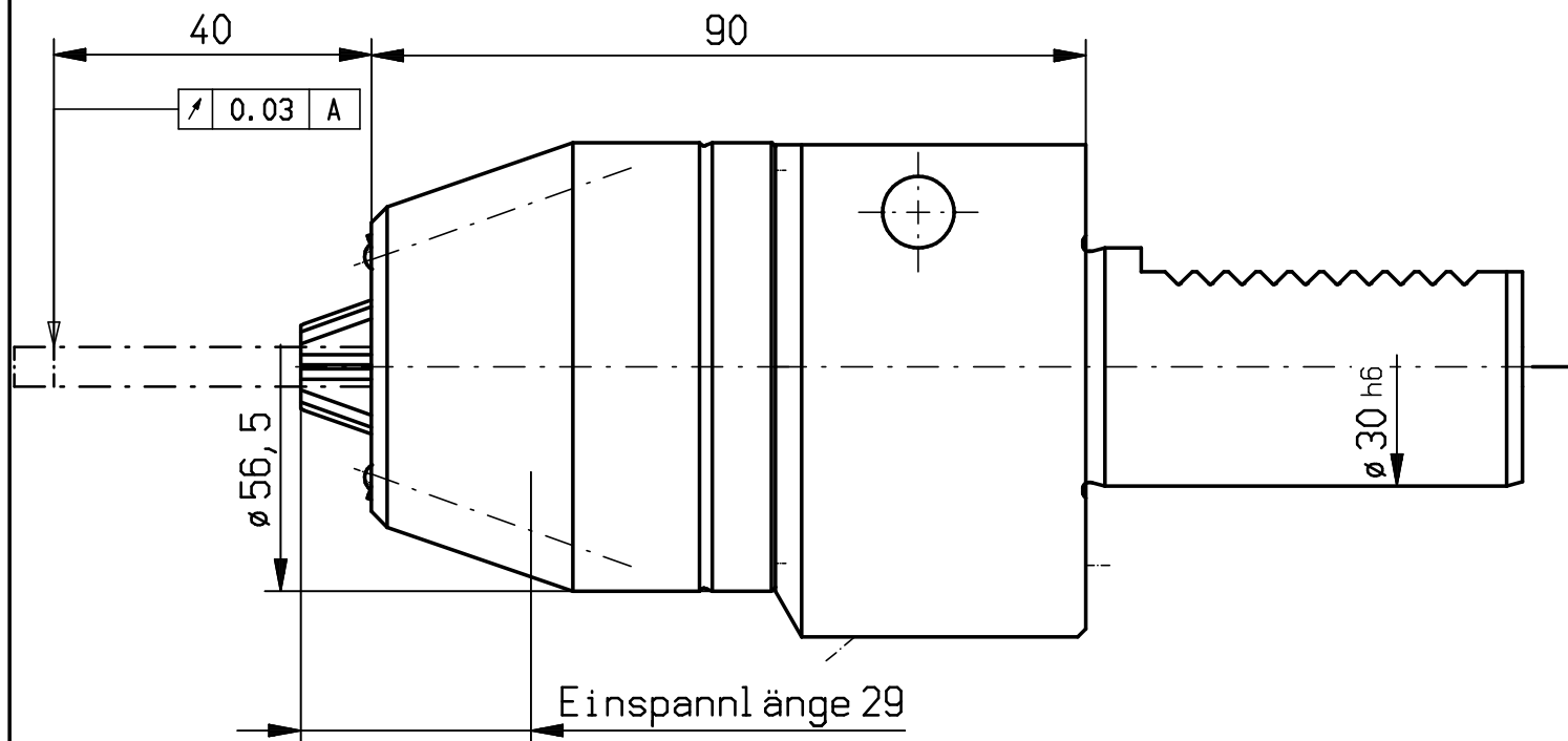
Ansicht Z M 1:1
